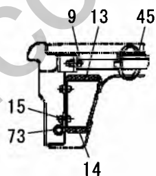
断面 Section C-C
