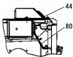
断面 Section B-B
